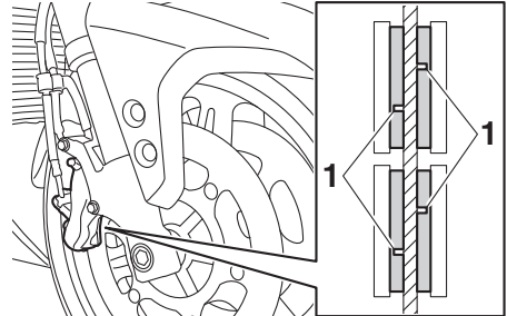
1. Verschleißanzeigergrille des Bremsbelags
