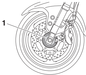
1. Vorderradnabe
