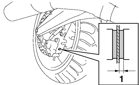
1. Bremsbelagstärke
