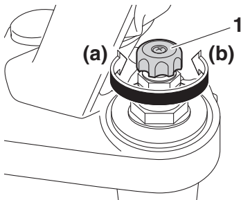
1. Zugstufendämpfungs-Einstellknopf
