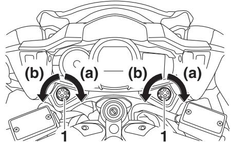
1. Scheinwerferkegel-Einstellknopf
