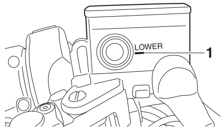
1. Minimalstand-Markierung
