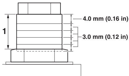
1. Abstand A
