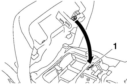
1. Zungenaufnahme "H"
