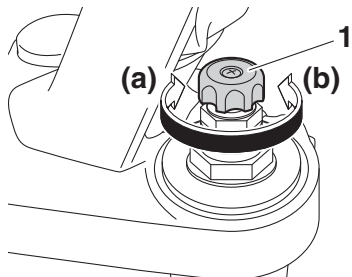
1. Zugstufendämpfungs-Einstellknopf
