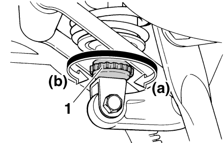
1. Zugstufendämpfungs-Einstellknopf
