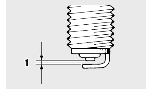
1. Zündkerzen-Elektrodenabstand
