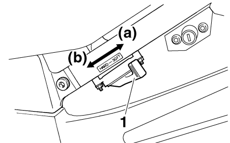
1. Einstellhebel der Federvorspannung
