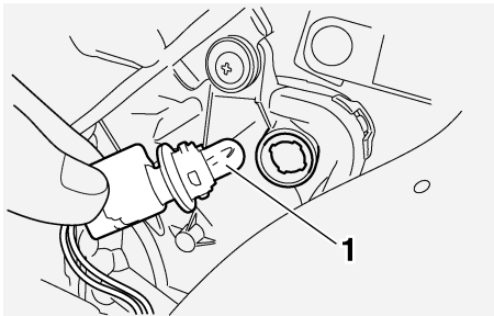
1. Standlichtlampe
