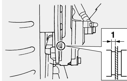
1. Bremsbelagstärke
